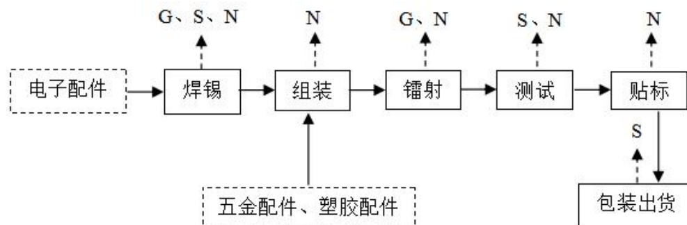
图 3-3 项目电子烟生产工艺及产污环节流程图
