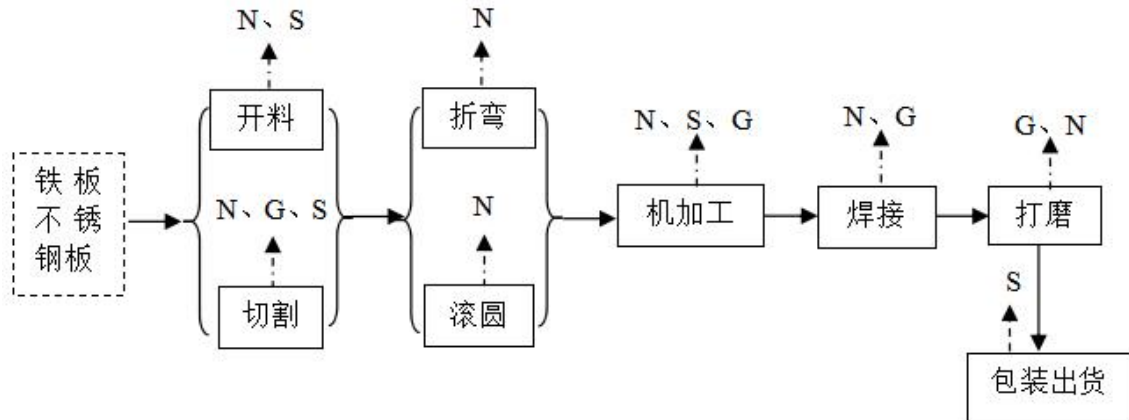
图 3-3 项目五金配件生产工艺及产污环节流程图
