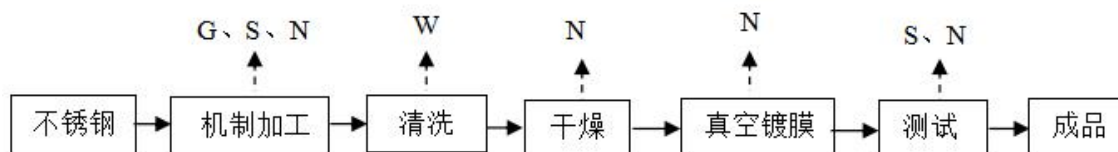
图 3-2 手表配件生产工艺及产污环节图
