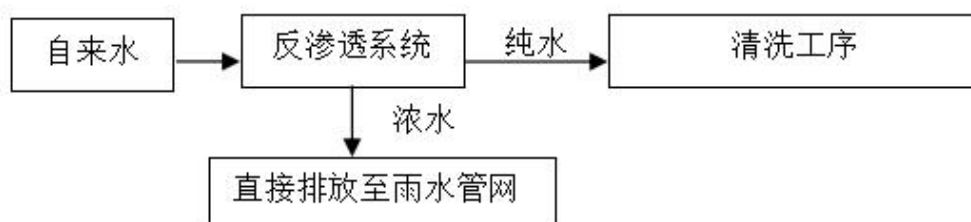
图 3-3 纯水制备生产工艺及产污环节图
