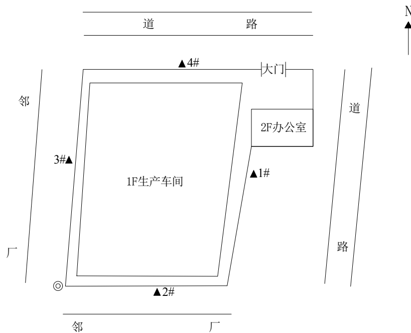
图 3-2 厂区平面布置及监测点位
